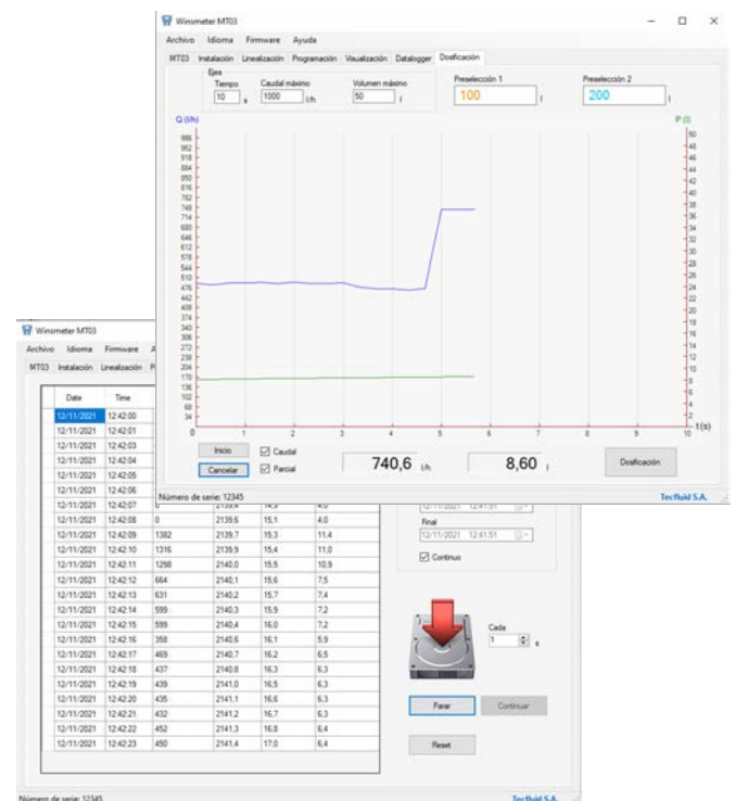
Convertidor MT03F
