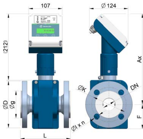
Convertidor XT5 montaje compacto
