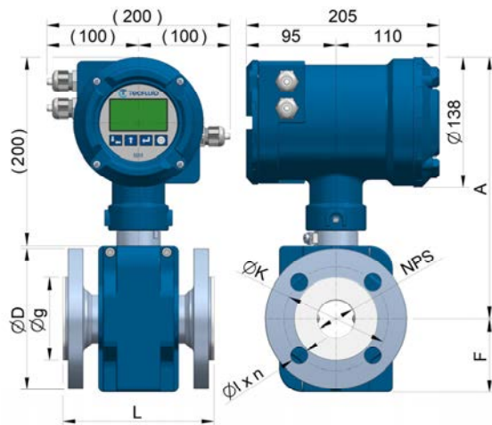
Convertidor XT5 montaje compacto
