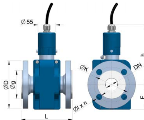
Convertidor montaje remoto
